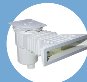
Skimmer Öffnung 50 cm breit, 8 cm hoch
