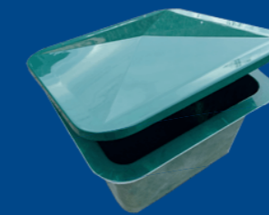
Technikschacht L x B x T: 100 cm x 100 cm x 70/85 cm + 9 cm Rand, mit Deckel
